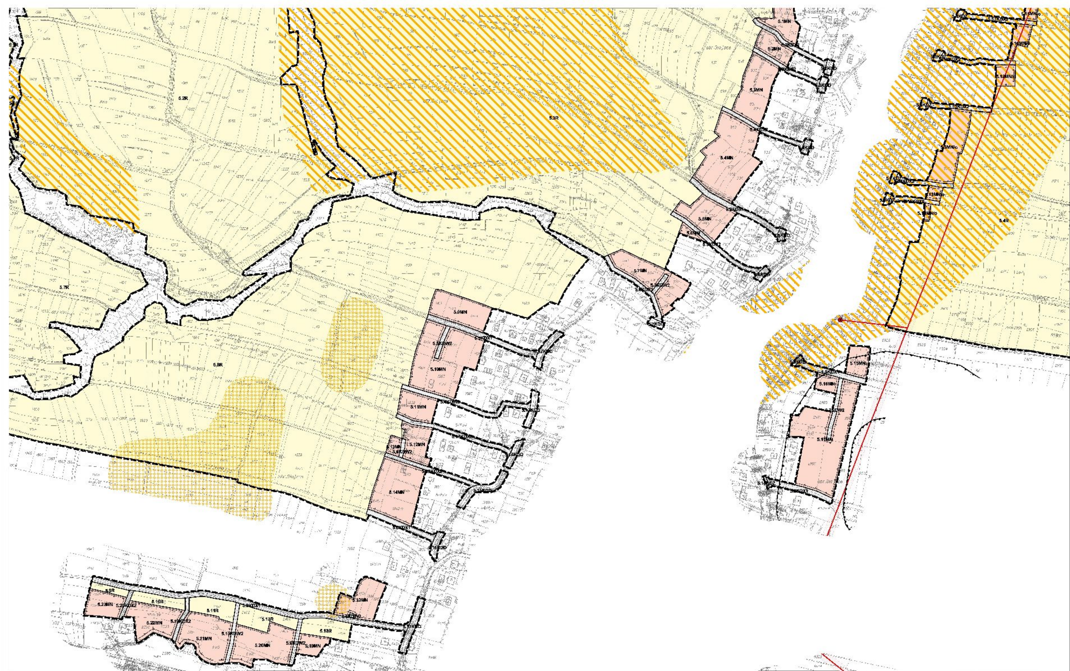
MIEJSCOWY PLAN ZAGOSPODAROWANIA PRZESTRZENNEGO CHYROWA GŁOJŚCE IWLA - 2 ZAŁĄCZNIK NR 1 DO UCHWAŁY NR .../... RADY MIEJSKIEJ W DUKLI Z DNIA ..... 2016 ROKU RYSUNEK PLANU - ARKUSZ NR 6 SKALA 1 : 2000
